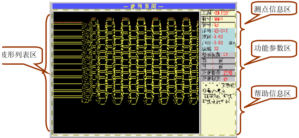
图 2.25 波列界面
