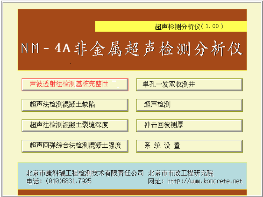
图 1.2 系统主界面
