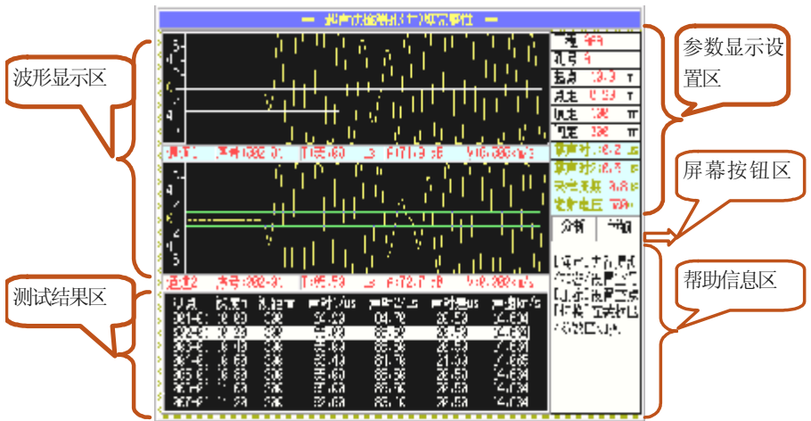
图 6.1 测井主界面
