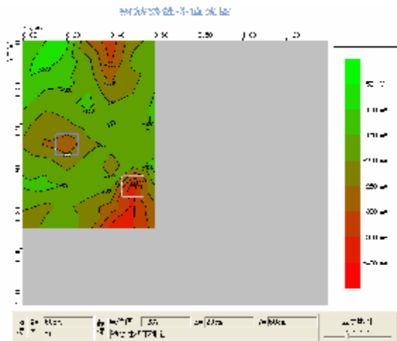
图 4.24 等值线图
