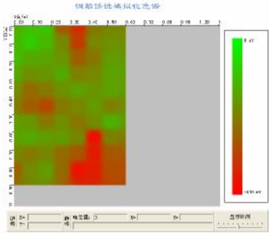
图 4.28 模拟化色谱
