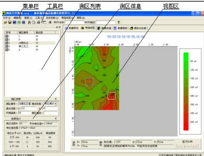
图 4.7 软件界面
