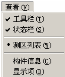
图 4.15 查看菜单
