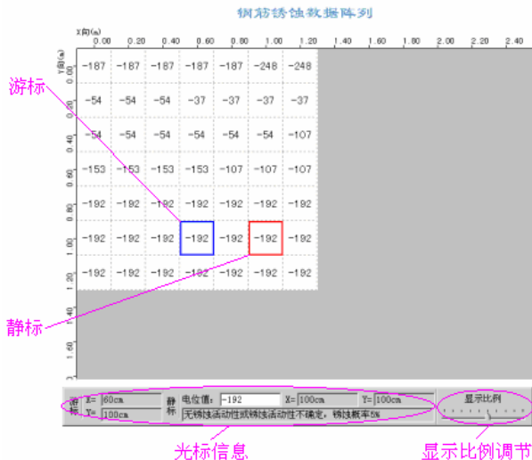
图 4.22 数据阵列
