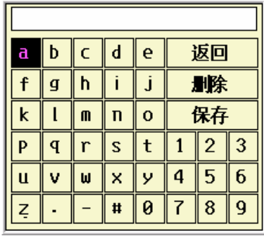
图 5.3 字符软键盘
