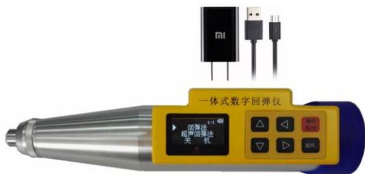
图 2-1 仪器组成
